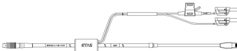
이더넷 PC 커넥션 및 전원 공급 케이블, Power Feeder는 PC에 근접, Lemo 1B FGL - RJ45 - Safety CBEP4155.1-5 F-00K-110-027 Banana (8fc-8mc+2mc), 5 m
