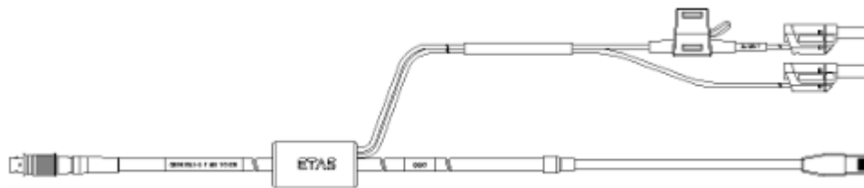
이더넷 PC 커넥션 및 전원 공급 케이블, Power Feeder는 PC에 근접, Lemo 1B FGL - RJ45 - Banana CBEP415.1-5 F-00K-105-680 (8fc-8mc+2mc), 5 m
