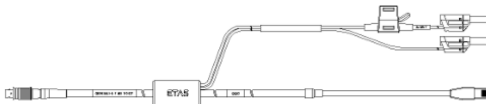
イーサネットPC 接続/ 電源ケーブル、Lemo 1B FGL - RJ45 - Safety Banana (8fc-8mc+2mc)、5m CBEP4155.1-5 F-00K-110-027
