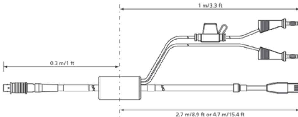
イーサネットPC 接続/ 電源ケーブル、Lemo 1B FGL - RJ45 - Safety Banana (8fc-8mc+2mc)、3m CBEP4105.1-3 F-00K-110-026
