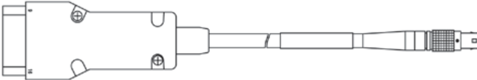
CAN 120 Ω 터미네이션 저항기, 2xDSUB CBCX131.1-0 F-00K-103-786 (9fc+9mc)
