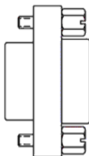
FlexRay 터미네이션 저항기 100 Ω, 2xDSUB (9fc-9mc) CBFX131.1-0 F-00K-104-689
