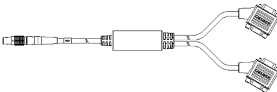
Abschlusswiderstand 100 \Omega , 2xDSUB (9fc-9mc)
