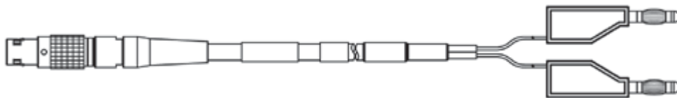
CAN-Schnittstellenkabel, DSUB - DSUB (9fc-9mc), 2 m
