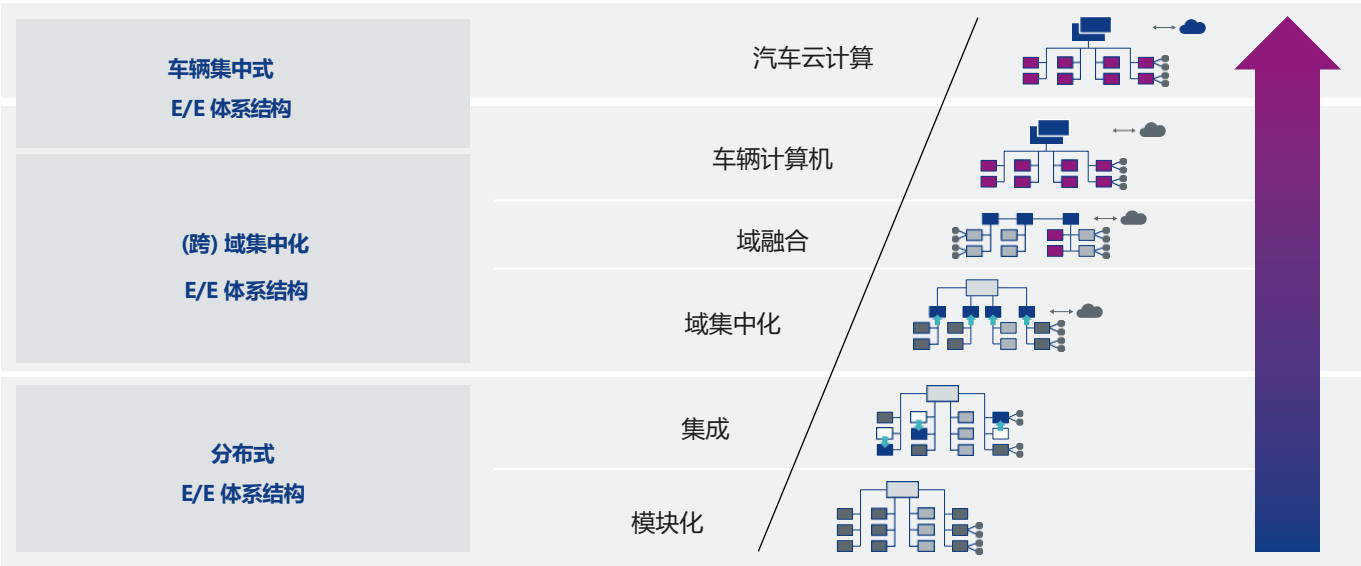
图 2: 车辆 E/E 架构从分布式到集中式的持续演变。
